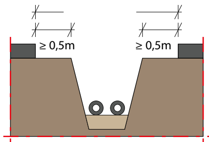
Asfaltin leikkausetäisyys reunan yli ajoradalla. Kuva.
