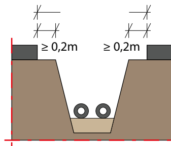
Asfaltin leikkausetäisyys reunan yli kevyenliikenteenväylillä. Kuva.
